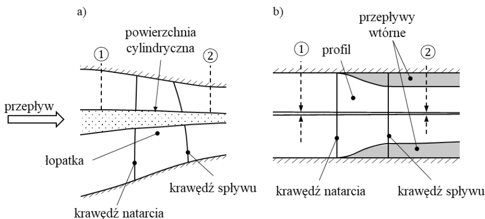
Rys. 1.9. Zmiana grubości strumienia w przepływie osiowym: a) przepływ przez sprężarkę osiową, b) przepływ przez palisadę liniową
