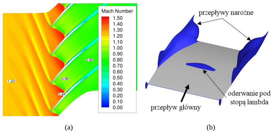
Rys. 4.5 Wyniki symulacji 3D: a) rozkład liczby Macha, b) wizualizacja przepływów wtórnych (obszar niebieski)
