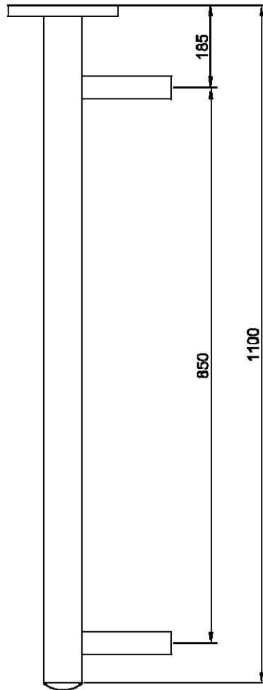
Rysunek 2 Schemat przyłącza bypass dla sondy z wariantu B
