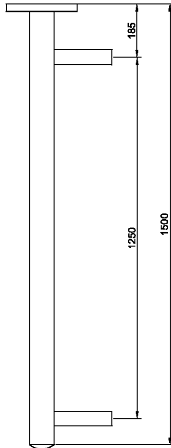
Rysunek 1 Schemat przyłącza bypass dla sondy z wariantu A
