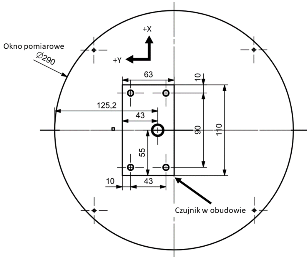
Rysunek 1 Schemat zamocowania czujnika do okna pomiarowego.
